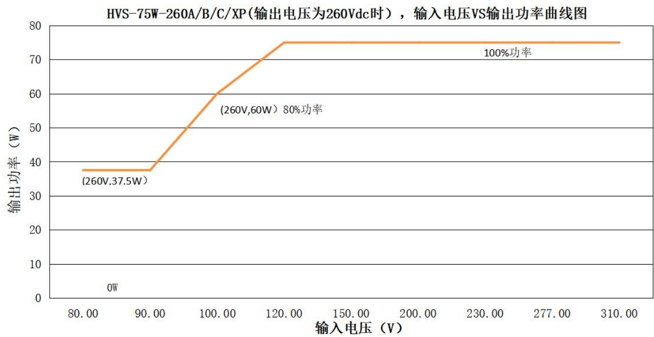
输出功率 VS 输入电压
