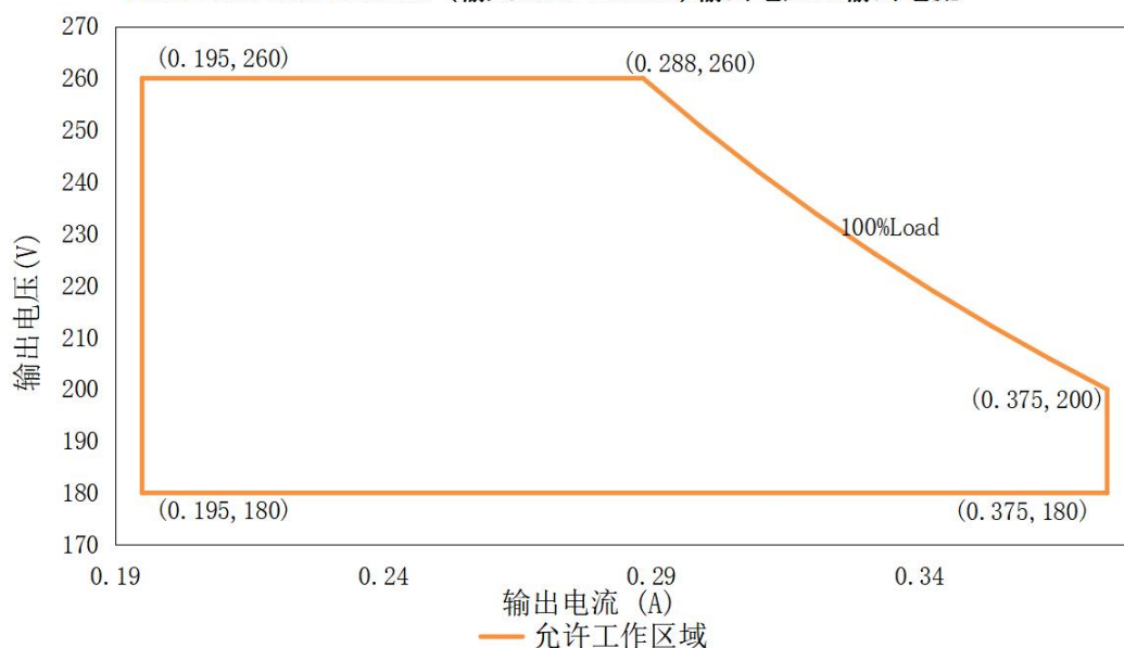
HVS-75W-260A/B/C/XP (输入: 100-277Vac) 输出电压VS输出电流
