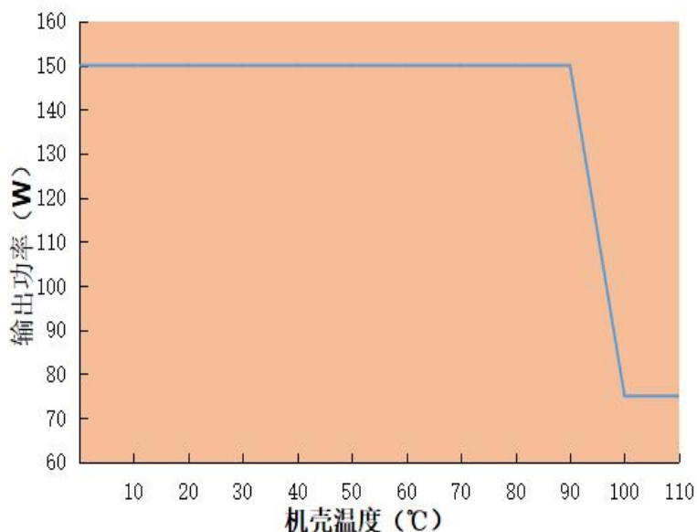
输出功率 VS 机壳温度
