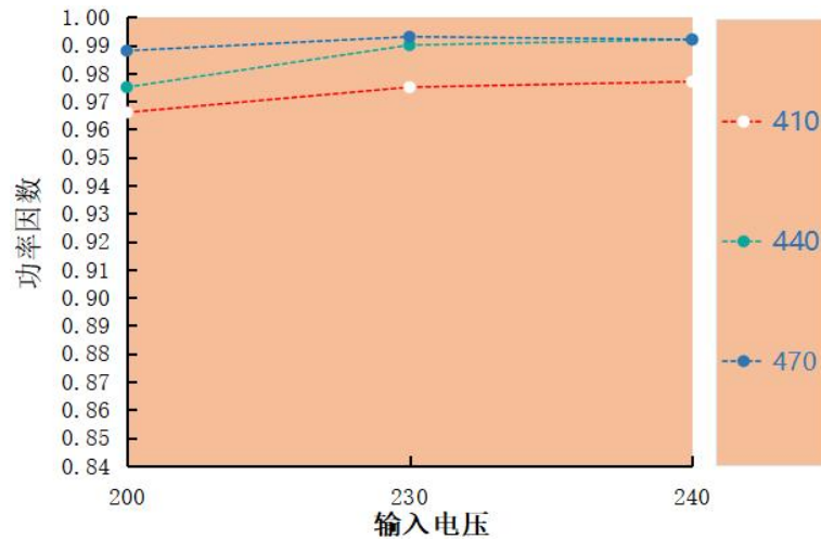
功率因素 VS 输入电压 LAS-120H-470A-XP
