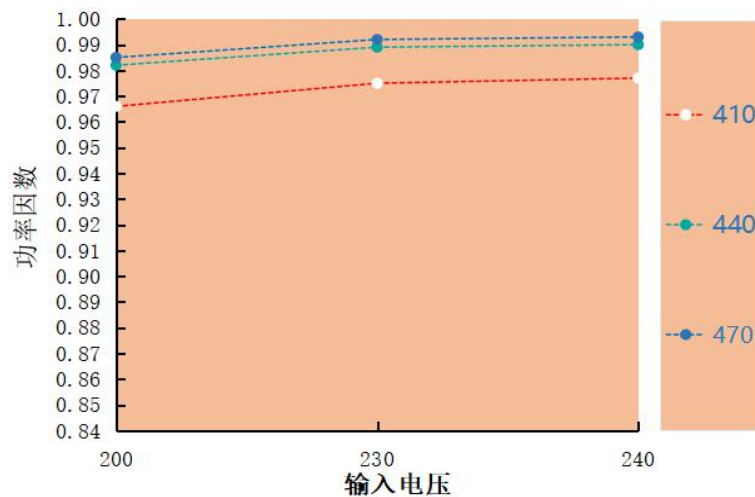
功率因素 VS 输入电压 LAS-120H-470A
