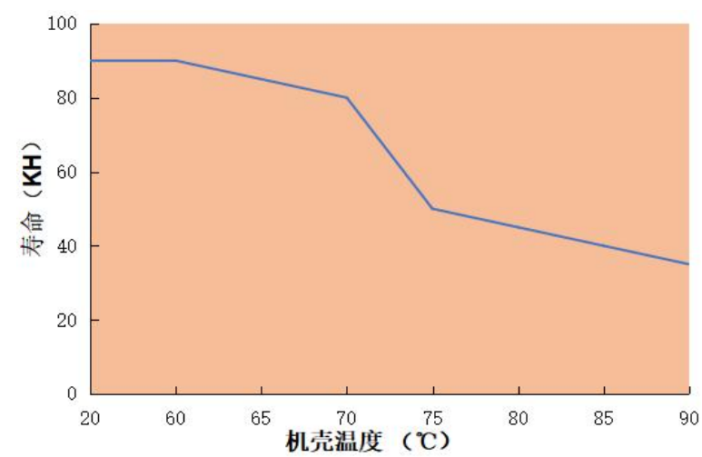
机壳温度 VS 寿命 LAS-120H-470A
