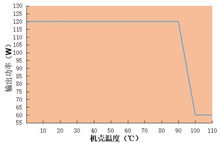
机壳温度 VS 输出功率 LAS-120H-470A-XP
