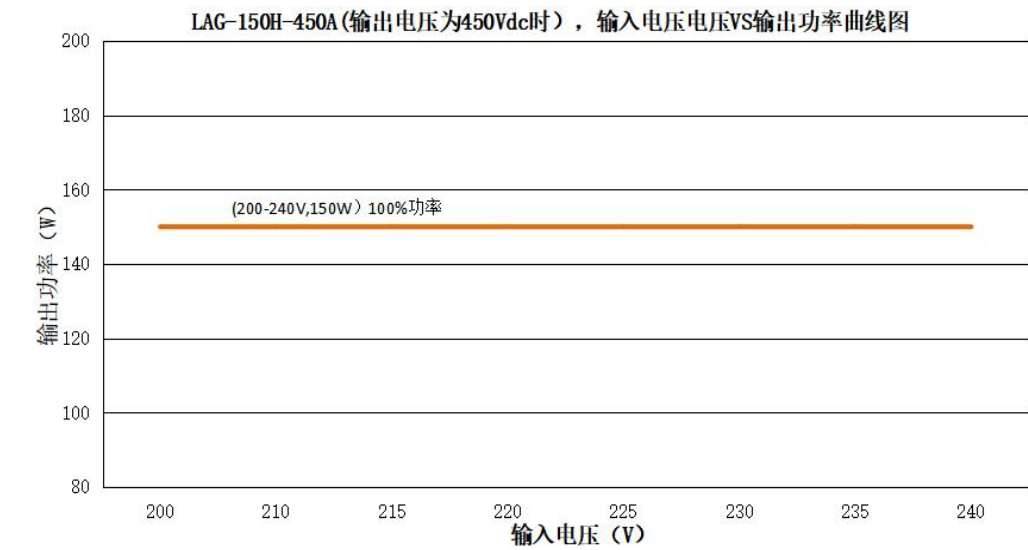
LAG-150H-450A(输出电压为 450Vdc 时，不同输入电压对应的额定输出电流值和输出功率)
