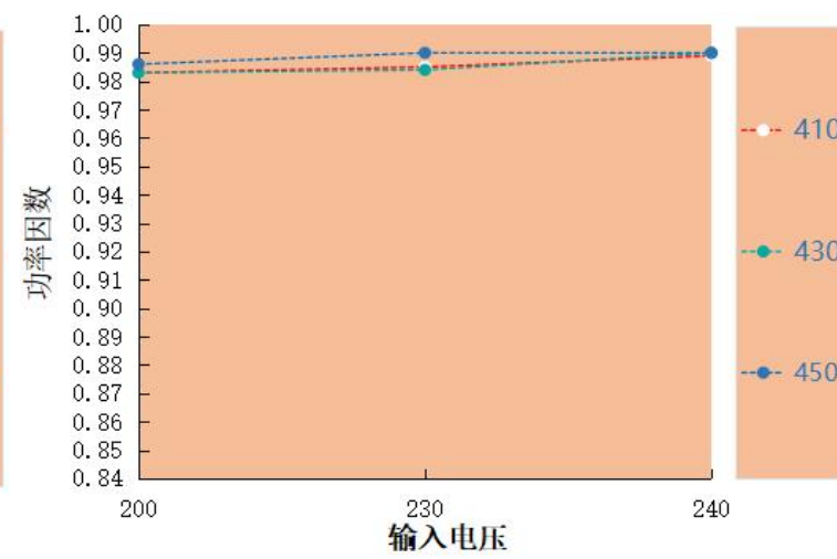
功率因素 VS 输入电压 LAG-150H-450A-XP
