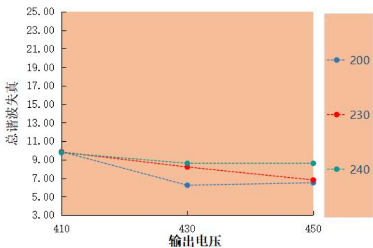
总谐波失真 VS 输出电压 LAG-150H-450A
