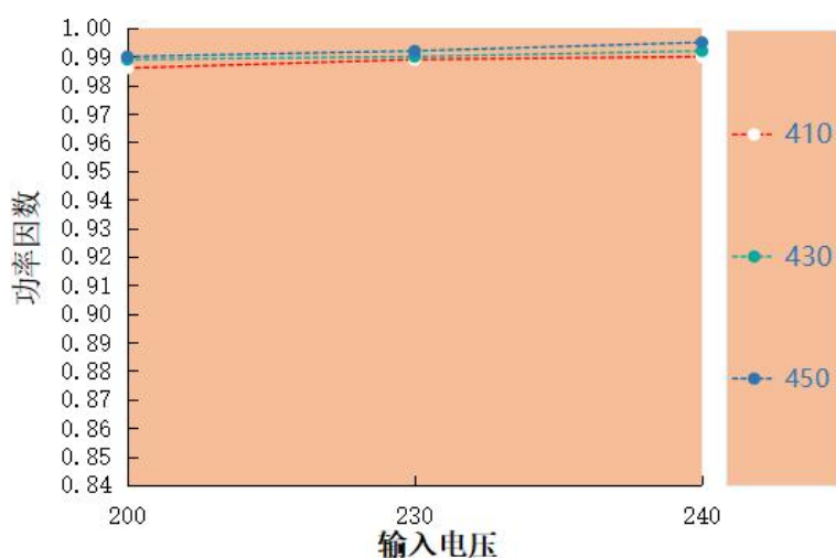
功率因素 VS 输入电压 LAG-150H-450A
