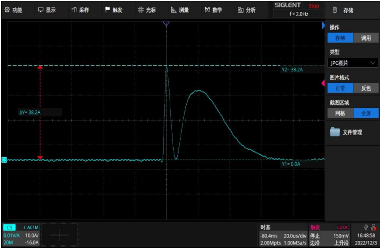
Surge curve(LAG-150H-450A)
