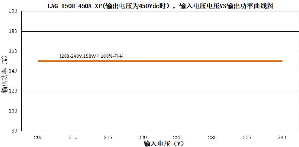
LAG-150H-450A-XP(输出电压为 450Vdc 时，不同输入电压对应的额定输出电流值和输出功率)
