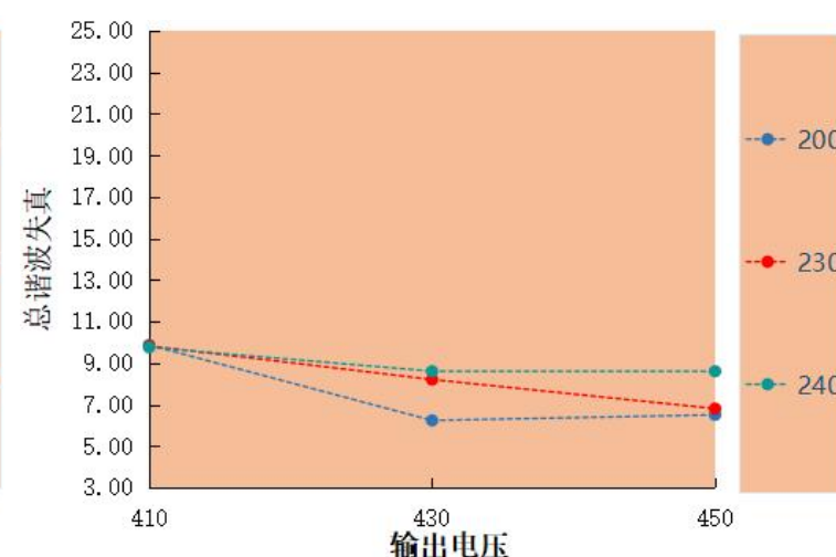
总谐波失真 VS 输出电压 LAG-150H-450A-XP
