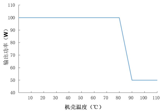
机壳温度 VS 输出功率
