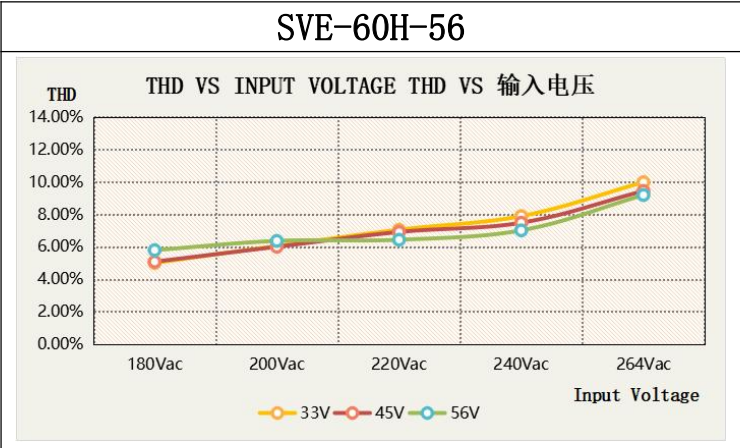
THD VS 输入电压
