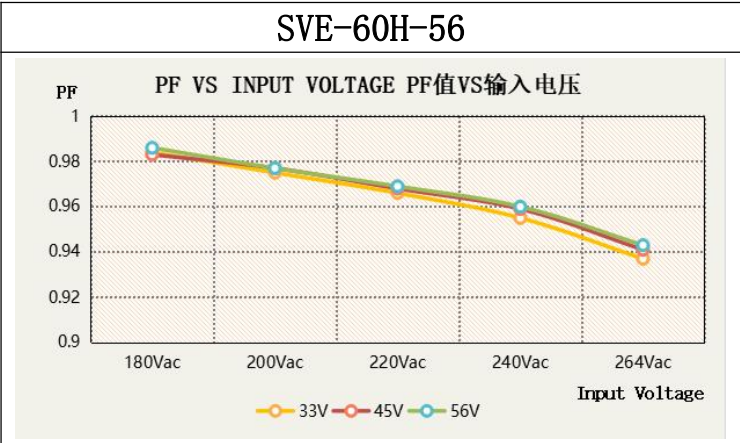
PF 值 VS 输入电压
