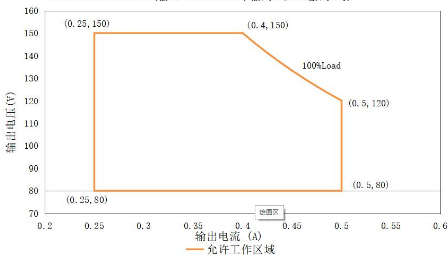
LBS-60W-150A/P/L (输入: 100-277Vac) 输出电压VS输出电流
